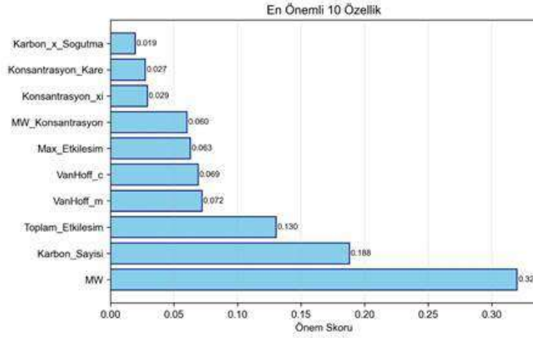
Şekil 2. Özellik önem analizine göre kritik parametrelerinin sıralanması
