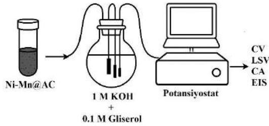
Şekil 1. Elektrokimyasal deneylerin yürütüldüğü sistem
