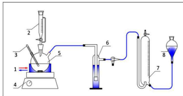
Şekil 1: Deney düzeneğinin şematik diyagramı.
