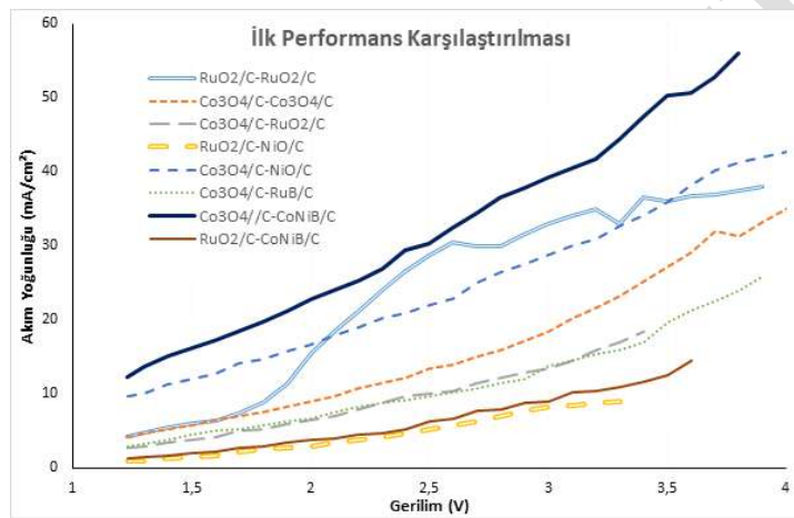
Şekil 3. MEA'ların ilk performanslarının karşılaştırması
