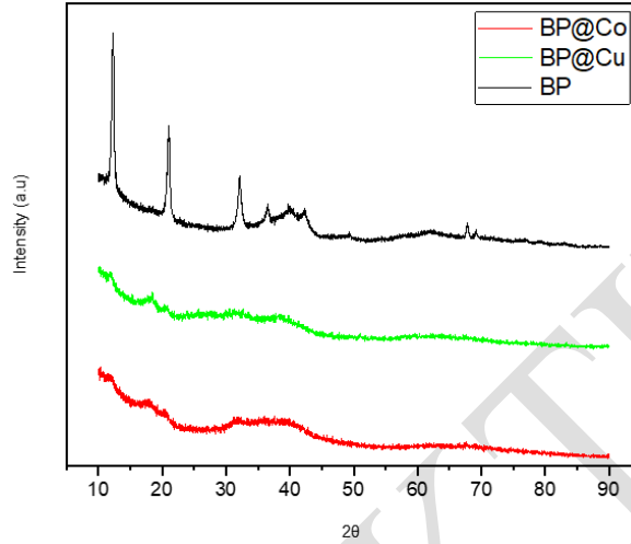
Şekil 1. BP, BP@Co ve BP@Cu yapılarına ait XRD sonuçları
