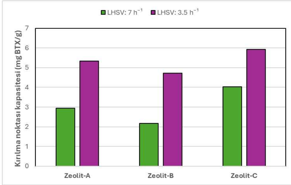
Şekil 1. Özel amaçlı üretilen farklı zeolit tiplerinin BTX kırılma noktası kapasiteleri
