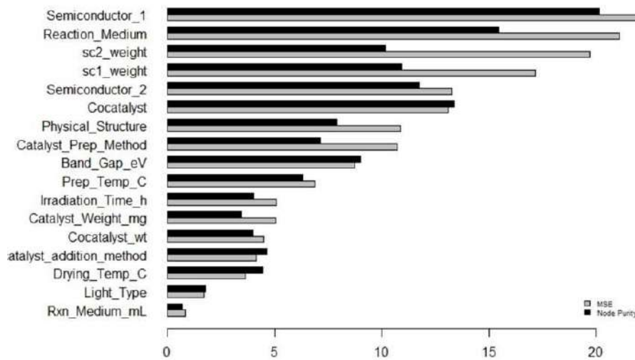
Şekil 2. Hidrojen üretimi için önem analizi.
