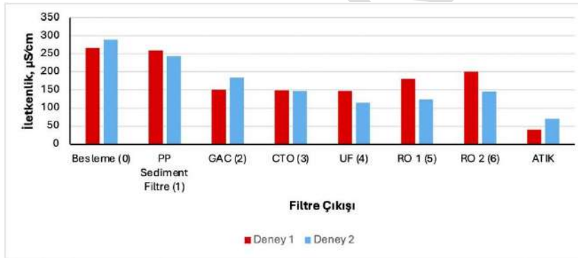
Şekil 6. Deney1 ve Deney2'nin karşılaştırmalı iletkenlik analizi
