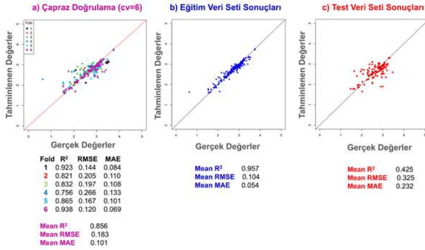
Şekil 2. İndirgenmiş (renkli) TiO 2 üretimi için RF modeli ile bant aralığı değerleri tahminlemesi için a) çapraz doğrulama, b) eğitim veri seti ve c) test veri seti sonuçları
