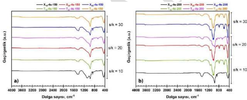
Şekil 2. Farklı parametreler ile sentezlenen malzemelerin kalsinasyon öncesi FTIR spektrumları
