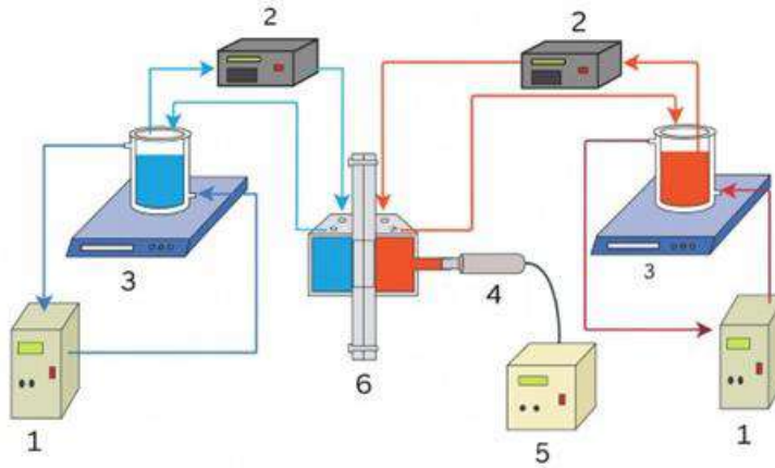
Şekil 1. Ultrases destekli DTMD konfigürasyonu (1: Isı değiştirici sirkülatörler, 2: Peristaltik pompalar, 3: Hassas teraziler, 4: Ultrasonik prob, 5: Ultrasonik homojenizatör, 6: Membran hücresi) [7]
