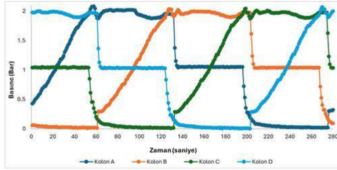
Şekil 3. PSA sisteminin basınç profili: Döngüsel kolon çalışması
