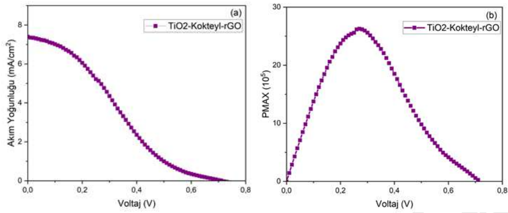
Şekil 1: TiO2- Kokteyl-(rGO) BDGH'sinin a) J-V b) Pmax-V grafiği
