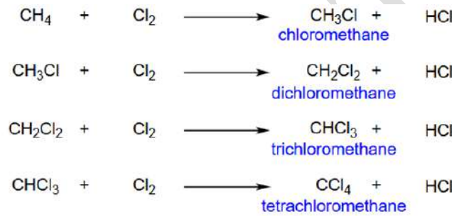
Şekil 2. Metan Klorinasyonu [5]
