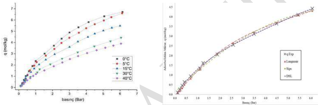
Şekil 1. Ticari Aktif Karbon Kullanılarak CO 2 Adsorpsiyon İzotermi ve İzoterm Modeli Uygunluk Sonuçları
