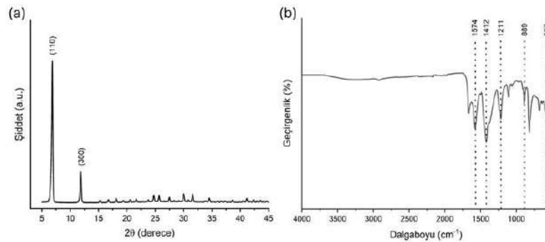
Şekil 2. Sentezlenen MOF'un a) XRD deseni ve b) FT-IR spektrumu
