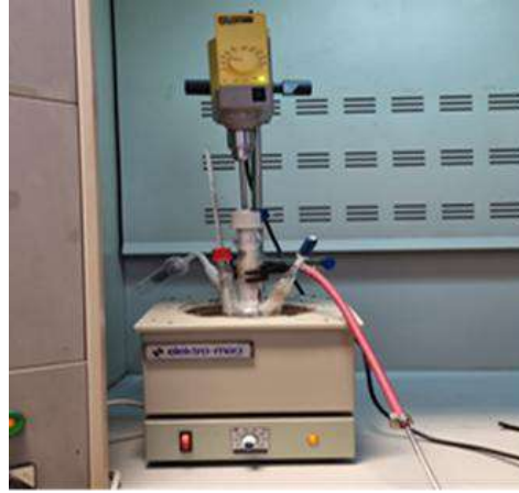
Şekil 1. PBI Sentezi deney düzeneği
