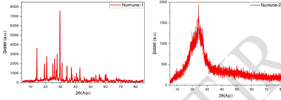
Şekil 3. Numune-1 ve Numune-2'nin XRD Grafiği
