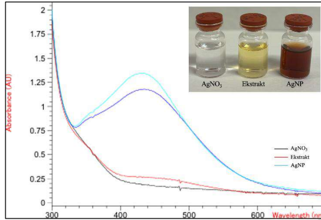
Şekil 1. AgNO 3 , Erica Arborea Ekstraktı ve AgNP 'nin UV-Vis Absorpsiyon Spektrumları
