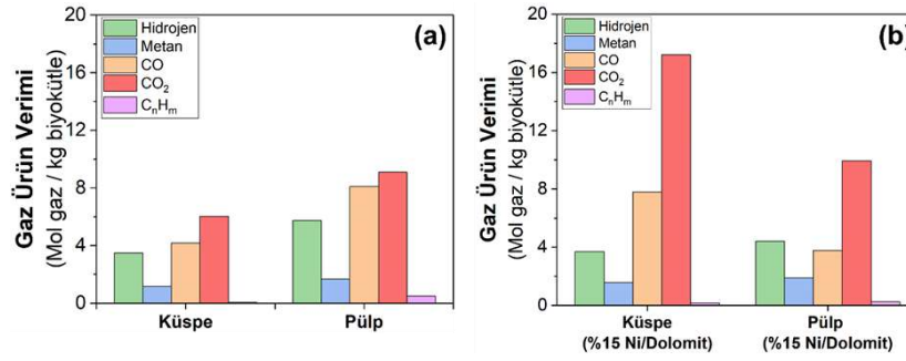
Şekil 3. Küşpe ve pülüpün (a) katalizörsüz ortamda (800 °C, 2 L/h hava besleme hızı) ve (b) %15 Ni/Dolomit varlığında (600 °C, 2 L/h hava besleme hızı, ağırlıkça %20 katalizör:biyokütle oranı) gazlaştırılmasından elde edilen gaz ürün verimleri
