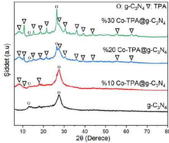
Şekil 2. g-C 3 N 4 , %10 Co-TPA@g-C 3 N 4 , %20 Co-TPA@g-C 3 N 4 ve %30 Co-TPA@g-C 3 N 4 'ün XRD desenleri.
