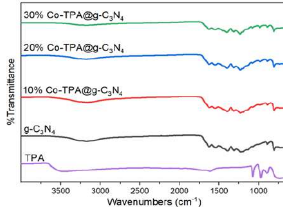
Şekil 1. TPA, g-C 3 N 4 ve farklı Co-TPA tuzu yüklemelerine sahip Co-TPA@g-C 3 N 4 nanokompozitlerinin FT-IR spektrumu.
