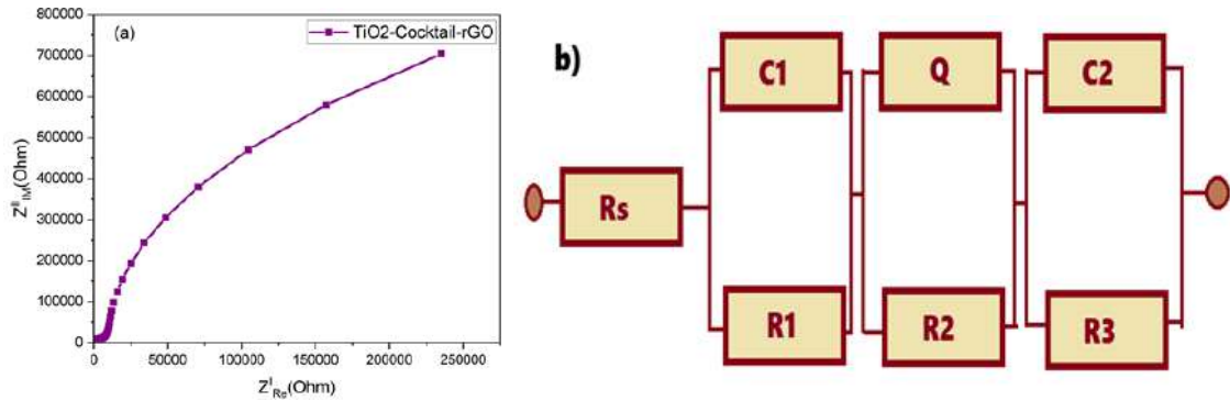
Şekil 3: TiO 2 -Kokteyl-rGO BDGH'sinin a) Nyquist diyagramı b) Devre Modeli
