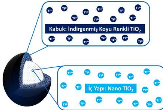
Şekil 1. İndirgenmiş renkli nano TiO 2 kabuk-çekirdek yapısının gösterimi
