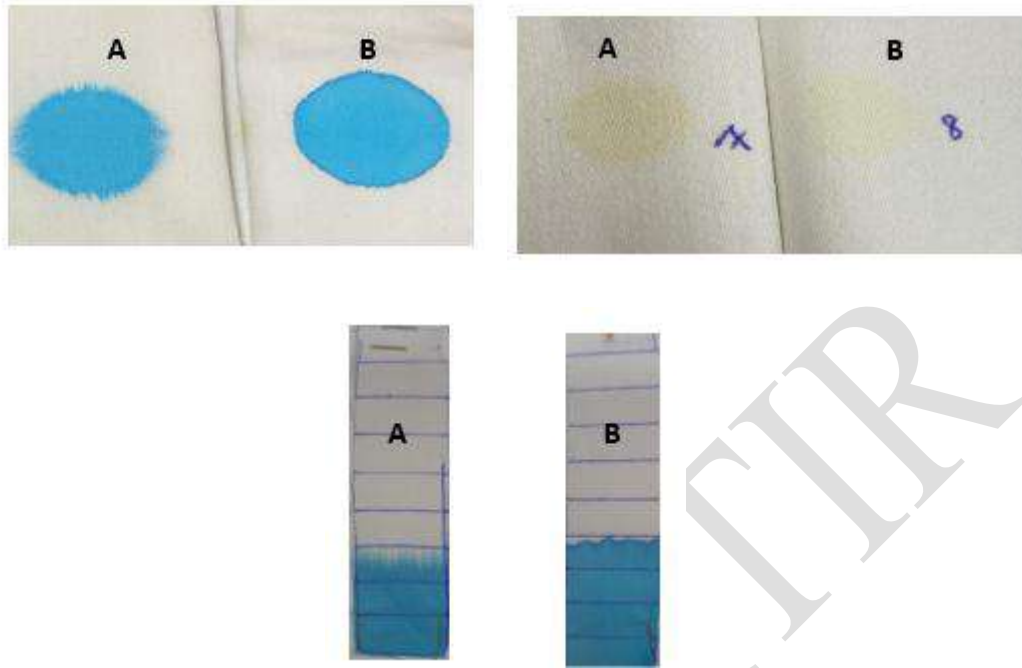
Şekil 1. Damlatma hidrofilite, Tegewa ve Kapilarite test sonuç görselleri (A klasik yöntemi ; B ise Entegre prosesi göstermektedir).
