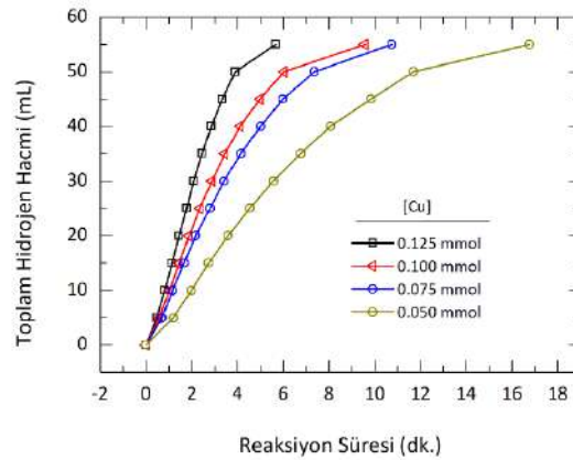
Şekil 2 - Cu/SiO 2 @Fe 3 O 4 katalizörü metal miktarına bağlı katalitik aktivite testleri
