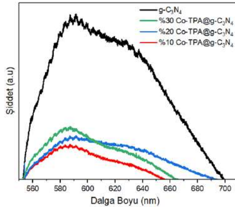
Şekil 4. g-C 3 N 4 , %10 Co-TPA@g-C 3 N 4 , %20 Co-TPA@g-C 3 N 4 , ve %30 Co-TPA@g-C 3 N 4 'ün PL spektrumları.
