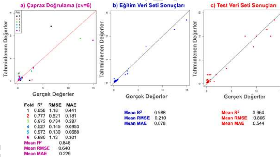
Şekil 5. İndirgenmiş (renkli) TiO 2 üretimi için XGBoost modeli ile olan XPS sonuçları eğrilerinin altında kalan alan üzerinden Ti 3+ (modifiye edilmiş ya da indirgenmiş TiO 2 ) / Ti 4+ (modifiye edilmemiş TiO 2 ) oranı tahminlemesi için a) çapraz doğrulama, b) eğitim veri seti ve c) test veri seti sonuçları
