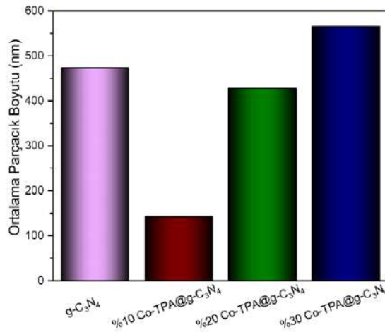
Şekil 5. g-C 3 N 4 , %10 Co-TPA@g-C 3 N 4 , %20 Co-TPA@g-C 3 N 4 ve %30 Co-TPA@g-C 3 N 4 'ün ortalama parçacık boyutu dağılımları.
