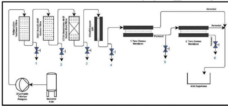
Şekil 1. Deney Sisteminin P&ID Diyagramı
