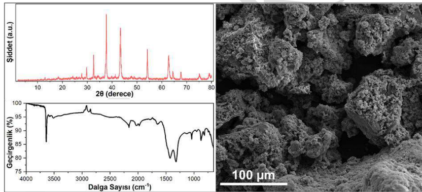
Şekil 2. Ağırlıkça %15 Nikel içeren Dolomit destekli katalizörün (a) XRD deseni, (b)FTIR spektrumu ve (c) SEM görüntüsü
