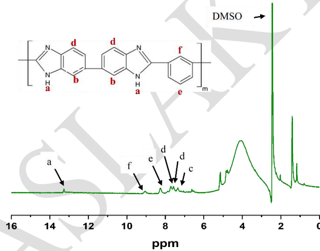
Şekil 5. Numune- 2'nin H-NMR spektrumu
