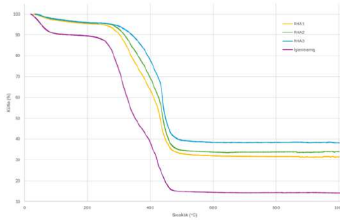
Şekil 2. İşlenmemiş pirinç kabuğunun, RHA 1, RHA 2, ve RHA 3'ün hava TGA eğrileri
