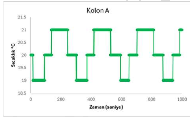
Şekil 4. PSA sisteminin sıcaklık profili: Döngüsel kolon çalışması
