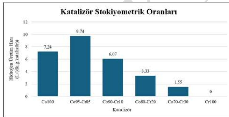
Şekil 2: Farklı stokiometrik oranlardaki katalizörlerin hidrojen üretim hızı değerleri.
