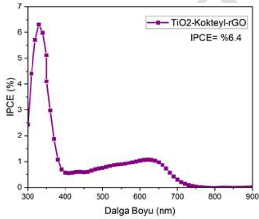
Şekil 2: TiO2-Kokteyl-rGO BDGH'sinin foton-akım dönüşüm verimi
