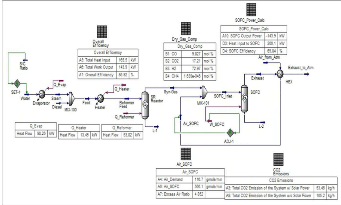
Şekil.1 Aspen HYSYS Modeli
