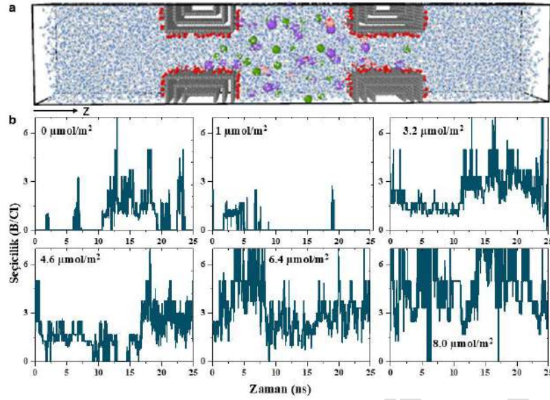
Şekil 1. Hidroksil Grubu Yüzey Yoğunluğunun CDI Elektrotlarında Borat Seçiciliğine Etkisi.
