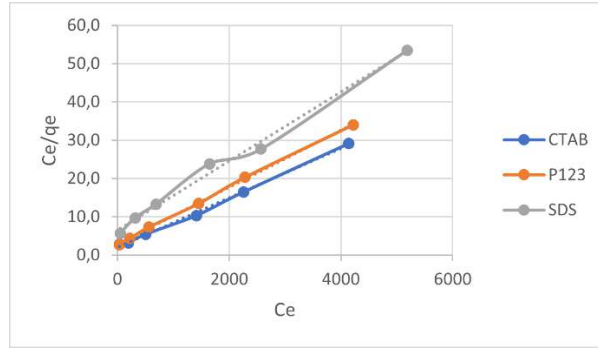
Şekil 2. Langmuir adsorpsiyonu izotermi linerarize grafik
