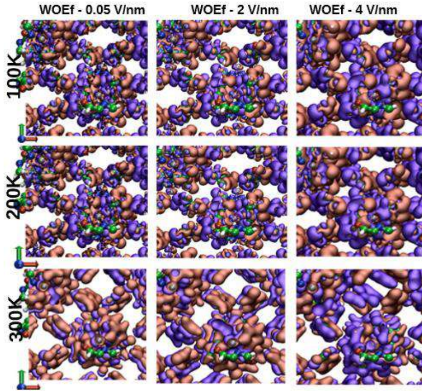
Şekil 4. Elektrik alan etkisiyle değişen, farklı sıcaklıklarda elektron yoğunluk farkı haritası.
