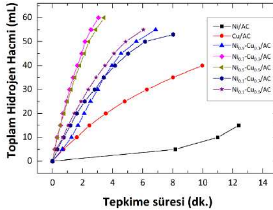
Şekil 1. Amonyak boranın hidroliz tepkimesinde, farklı mol oranlarına sahip Ni x Cu 1-x /AC katalizörlerinin hidrojen salınım hızına etkisi
