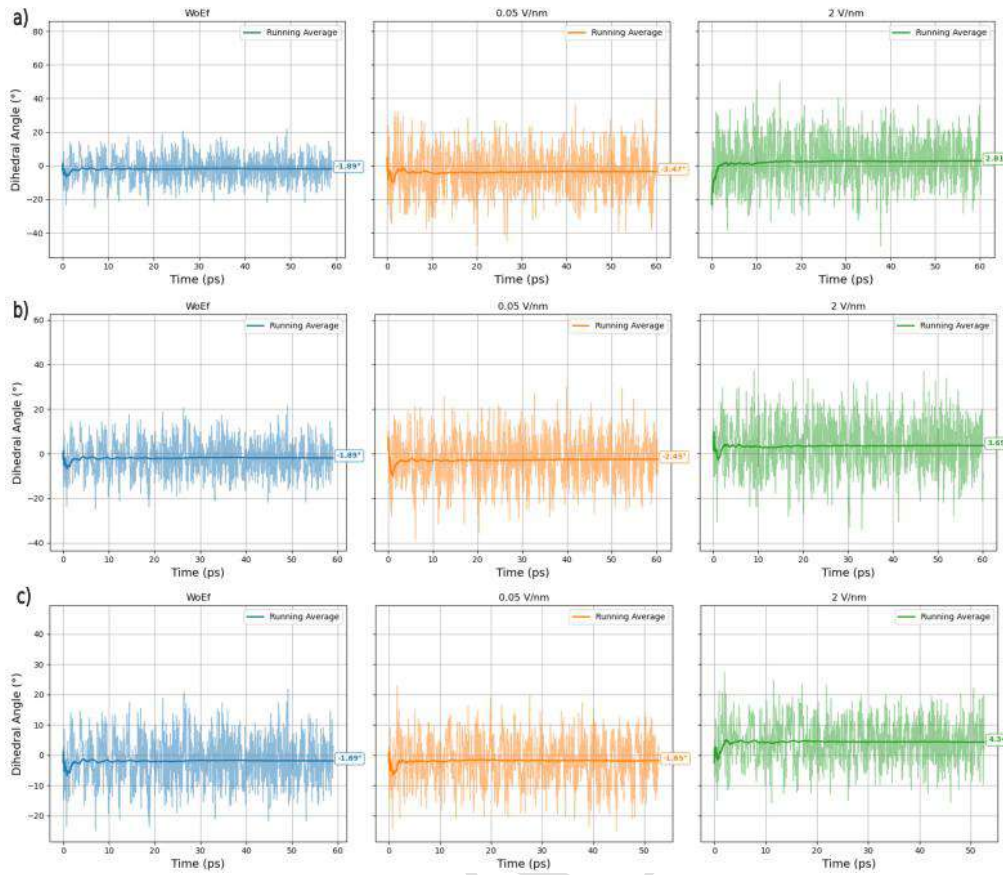
Şekil 2. Farklı sıcaklık ve elektrik alan şiddetlerinde ZIF-90 ligandlarının dihedral açı-zaman grafiği (AIMD sonuçları)
