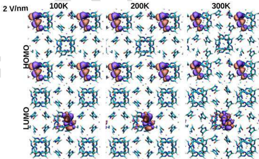
Şekil 3. 2 V/nm'de farklı sıcaklıklar için ZIF-90'ın HOMO–LUMO orbital dağılımı.
