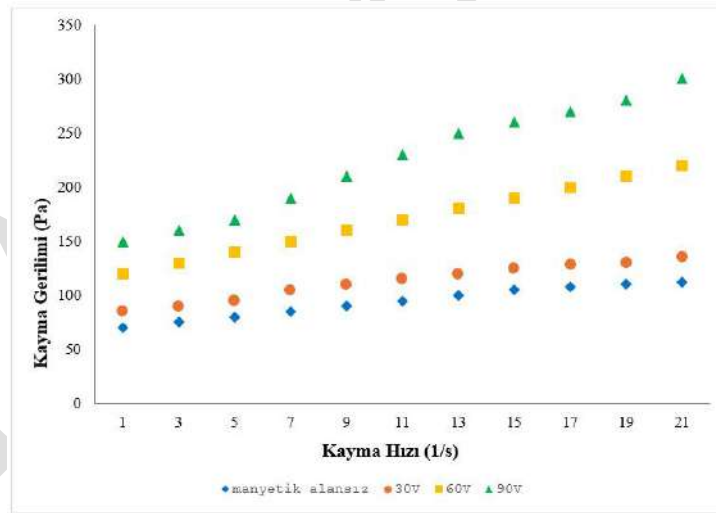
Şekil 2b. %30 oranında lazer yazıcı toner tozu içeren MR akışkanının reolojik davranışı
