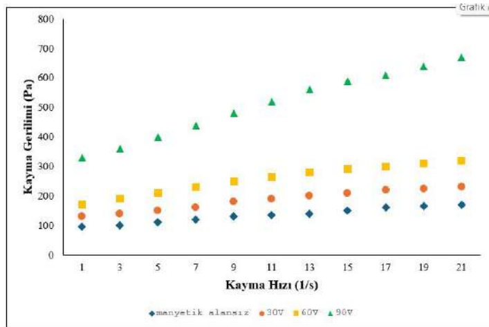
Şekil 2c. %45 oranında lazer yazıcı toner tozu içeren MR akışkanın reolojik davranışı
