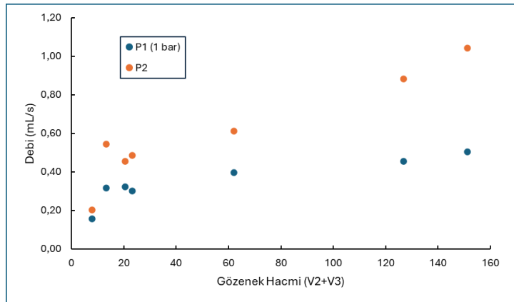
Şekil 5. Çıkış Debisinin Gözenek Boyutuna Göre Değişimi
