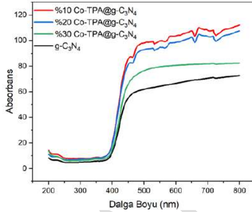
Şekil 3. g-C 3 N 4 , %10 Co-TPA@g-C 3 N 4 , %20 Co-TPA@g-C 3 N 4 , ve %30 Co-TPA@g-C 3 N 4 'ün UV-Vis DRS spektrumları.
