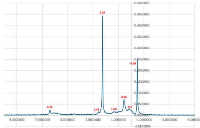
Şekil 4. C6D6 çözgeninde çözölmüş katran örneğinin 1H NMR sonuçları
