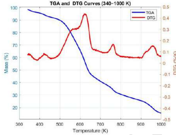
Şekil 1. Quercus vulcanica kabuğunun termogravimetri (TGA) ve diferansiyel termogravimetri (DTG) eğrileri
