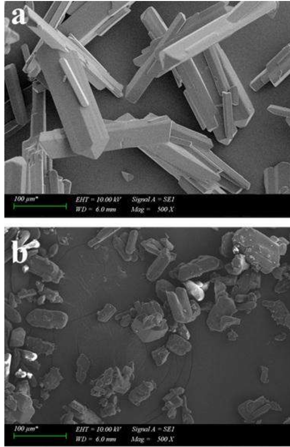
Şekil 1. a) Saf ortamda ve b) katkı maddesi varlığında elde edilen glisin kristallerinin SEM fotoğrafları.
