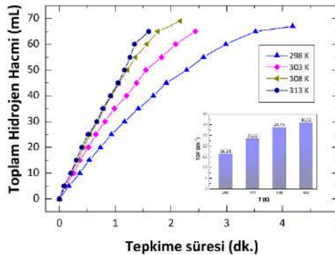
Şekil 2. Ni 0,7 Cu 0,3 /AC katalizörü için reaksiyon sıcaklığının hidrojen salınım hızına etkisi
