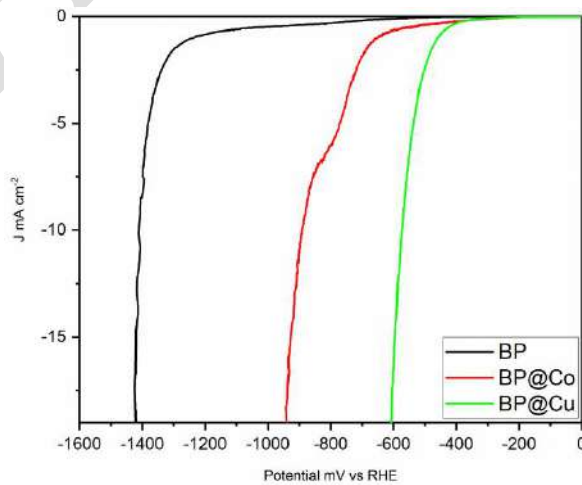
Şekil 2. BP, BP@Co ve BP@Cu yapılarına ait LSV sonuçları
