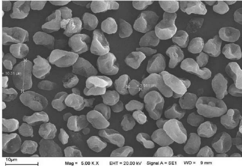
Şekil 1b. Farklı büyütme değerlerindeki lazer yazıcı toner tozunun SEM görüntüsü
