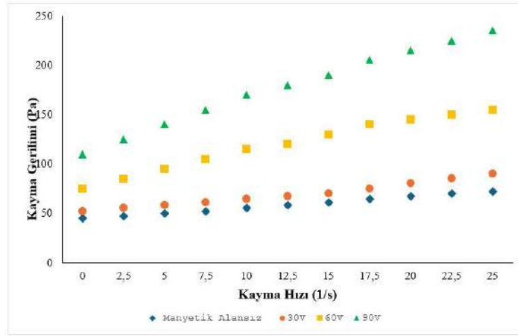
Şekil 2a. %15 oranında lazer yazıcı toner tozu içeren MR akışkanının reolojik davranışı
