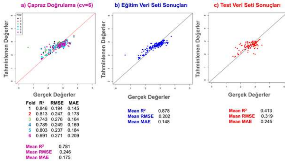
Şekil 3. İndirgenmiş (renkli) TiO 2 üretimi için XGBoost modeli ile bant aralığı değerleri tahminlemesi için a) çapraz doğrulama, b) eğitim veri seti ve c) test veri seti sonuçları
