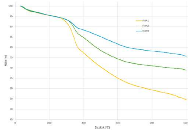
Şekil 3. RHA 1, RHA 2, ve RHA 3'ün argon TGA eğrileri
