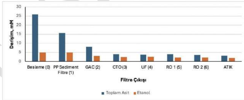
Şekil 4. Deney2'nin filtre çıkışlarındaki toplam asit derişimi ve etanol derişimi
