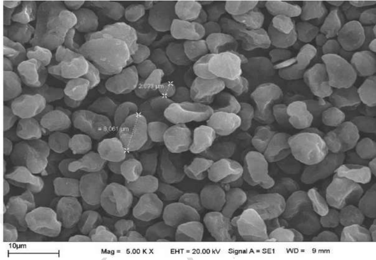
Şekil 1a. Farklı büyütme değerlerindeki lazer yazıcı toner tozunun SEM görüntüsü
