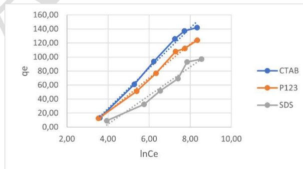
Şekil 4. Temkin adsorpsiyonu izotermi linerarize grafik
