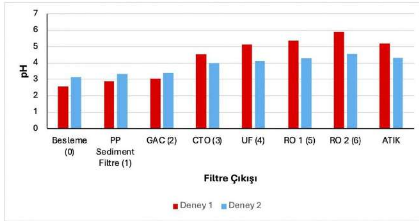
Şekil 5. Deney1 ve Deney2'nin karşılaştırmalı pH analizi
