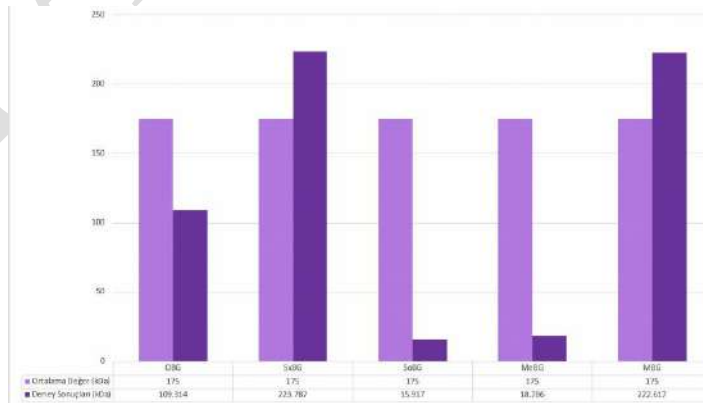
Şekil 1. Literatürde bildirilen ortalama beta gluklan molekül kütlesi değerleri [9] ile deneysel olarak elde edilen sonuçların örnekler bazında karşılaştırılması.
