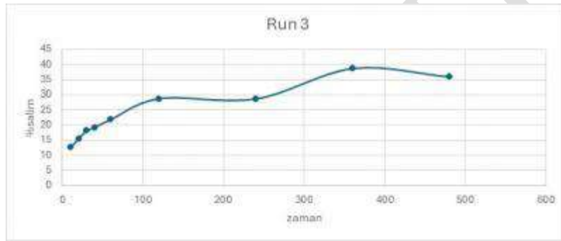
Şekil 1. Run 3 numunesi için quercetin salımının zamana bağlı değişim grafiği
