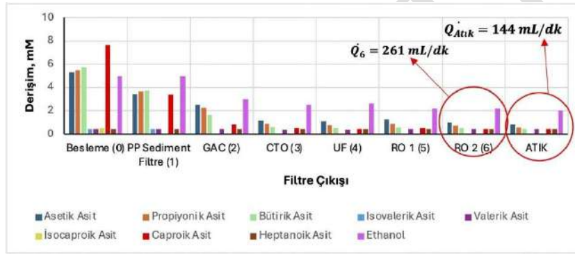
Şekil 3. Deney2'nin GC analiz sonuçları
