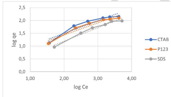
Şekil 3. Freundlich adsorpsiyonu izotermi linerarize grafik
