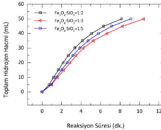
Şekil 1 – Amonyak boranın Cu/SiO 2 @Fe 3 O 4 katalizörü varlığında hidrolizinde Fe 3 O 4 :SiO 2 oranının hidrojen üretim hızına etkisi
