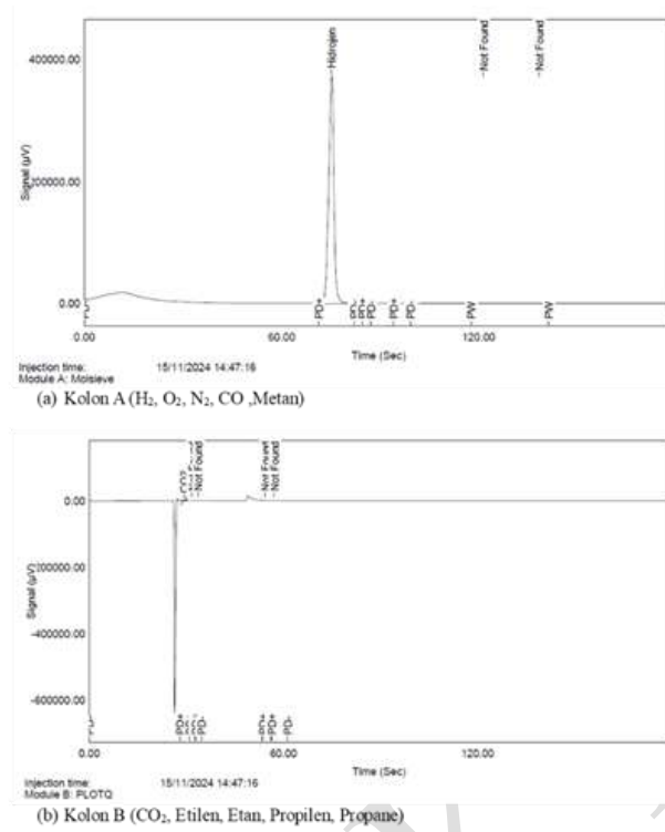
Şekil 6. Gaz Kromatografi Analizi sonuçları
