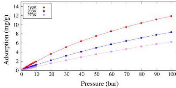
Şekil 1. ZIF-90'ın farklı sıcaklıklarda H_2 adsorpsiyon izotermi
