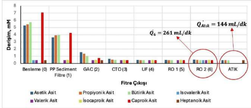
Şekil 2. Deney1'in GC analiz sonuçları
