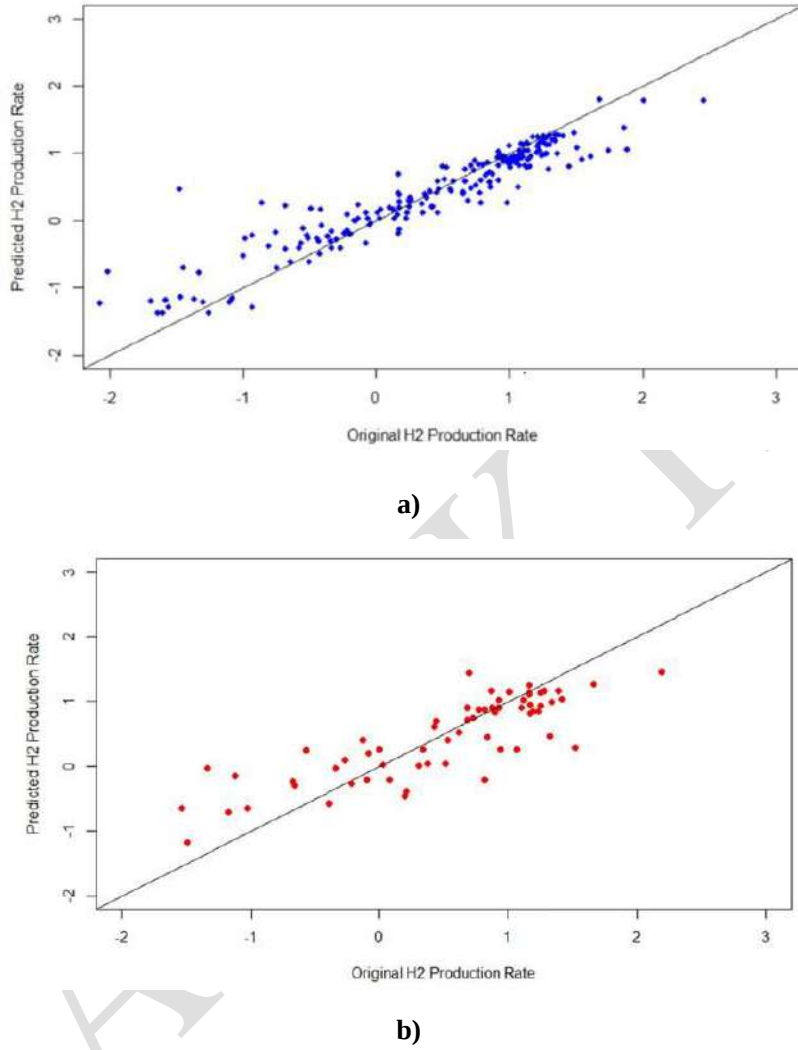
Şekil 1. Hidrojen üretimi için geliştirilen modeldeki a) eğitim seti b) test seti.
