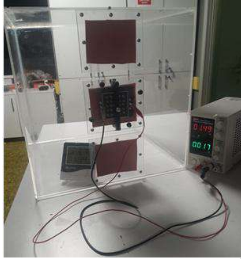
Şekil 2. MEA'ların ilk performans testi için deney düzeneği
