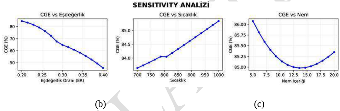
Şekil 3: CGE için sensitivity analiz (a) CGE vs Eşdeğerlik, (b) CGE vs Sıcaklık, (c) CGE vs Nem
